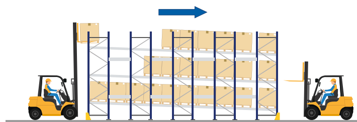
SISTEMA FIFO
